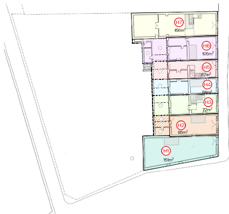
Planta baixa
