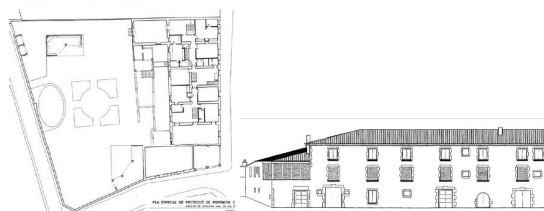
Planta i alçat de la finca de Can Mandri en el seu estat actual.
