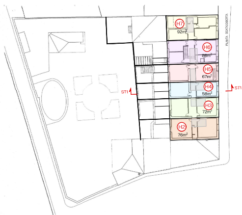
Planta sotacoberta
